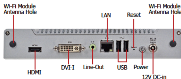
后面板
