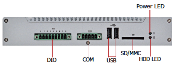
前面板
