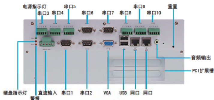
后面板 HICS 522-LRA060
