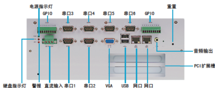
后面板 HICS 522-LR6G60
