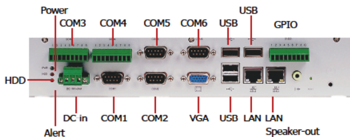
后面板
