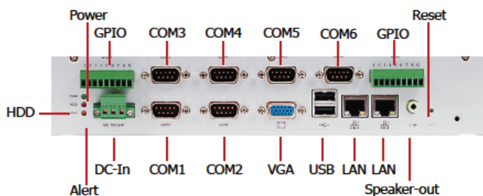
后面板
